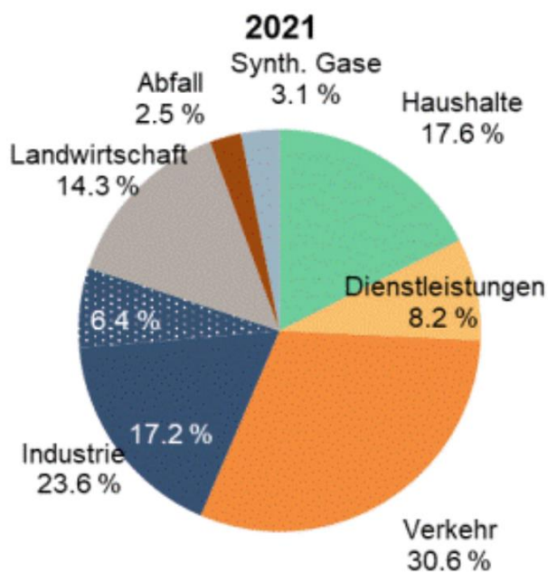
Abbildung 7: Anteile der Sektoren an den Treibhausgasemissionen innerhalb der Schweiz von insgesamt 45.3 Mio. t/CO 2 eq im Jahr 2021. Treibhausgas-Inventar Schweizer Landwirtschaft
