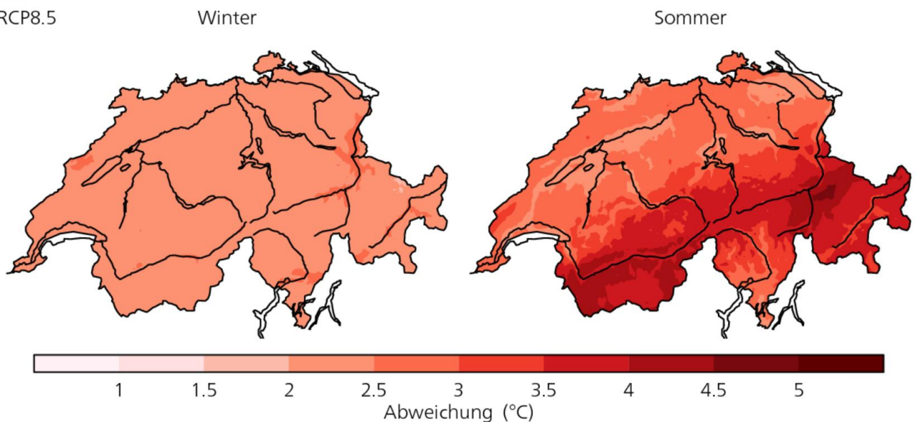
Abbildung 6: Temperaturrends im saisonalen Mittel für das Jahr 2060 ohne Klimaschutzmassnahmen (Emissionsszenario RCP8.5) (MeteoSchweiz, 2023)
